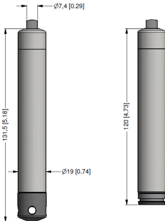
Fig. 22-3 Sonde – AquaBar BS
