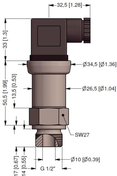
Fig. 22-1 Sonde - UniBar E II avec fiche
