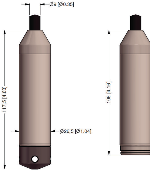
Fig. 22-4 Sonde – AquaBar II
