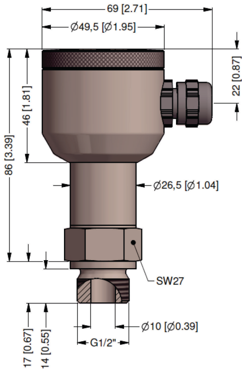
Fig. 22-2 UniBar E II avec écran (dans un boîtier en acier inoxydable)
