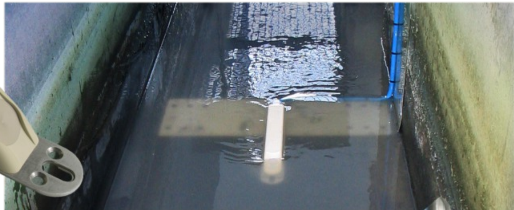
Capteur ultrason aérien pour la mesure de niveau, montage en voûte de conduite
